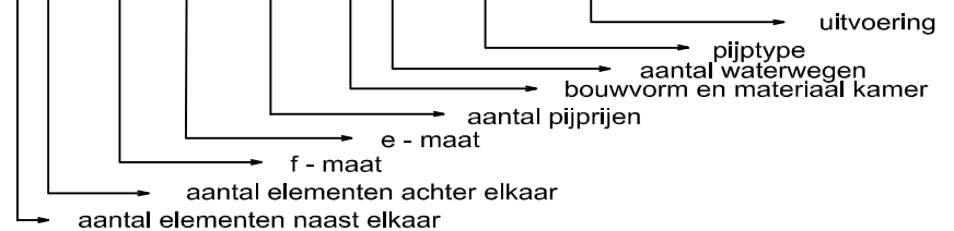
Zijwaardse uitvoering voor horizontale luchtstroom
